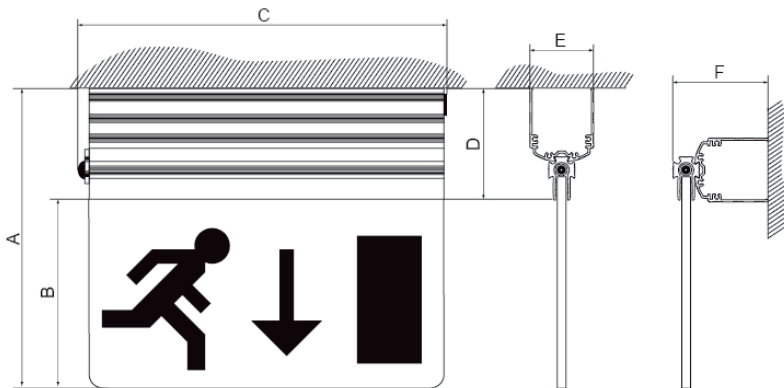
Dimensioner (mm)
